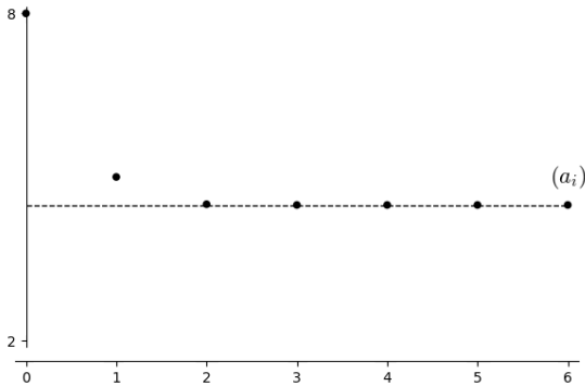
Obrázek 1.1: složka (a_i)
