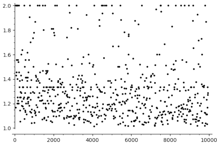
Obrázek 3.6: Číslo \frac{S(\mathbb{F}_p) \cdot (p-1)}{D(\mathbb{F}_p)} pro p < 10^4
