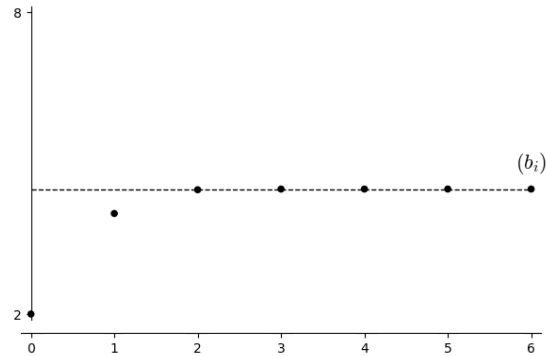
Obrázek 1.2: složka (b_i)
