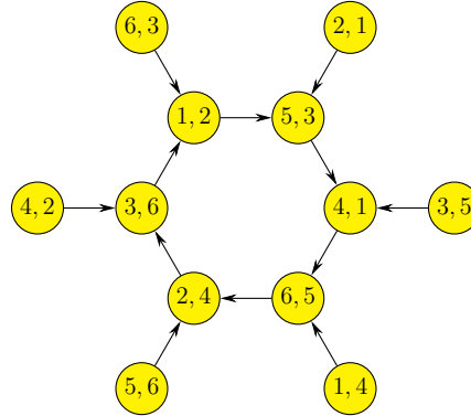
Obrázek 2.1: Roj AG_{\mathbb{F}_7} .
