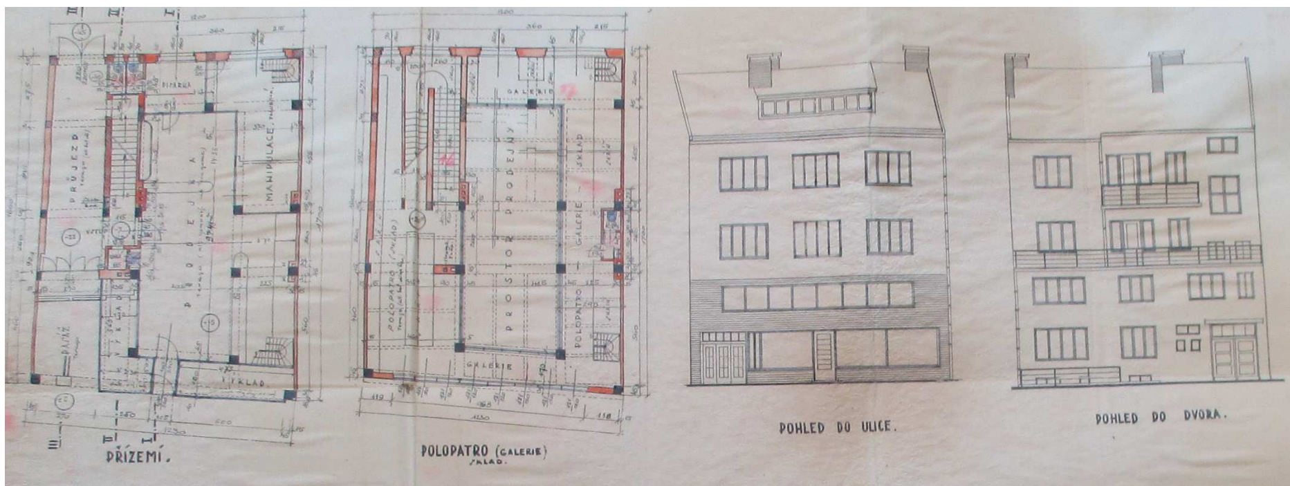
Obrázek č. 46: Výřez části stavebního plánu domu č. p. 6 na Žižkově náměstí
