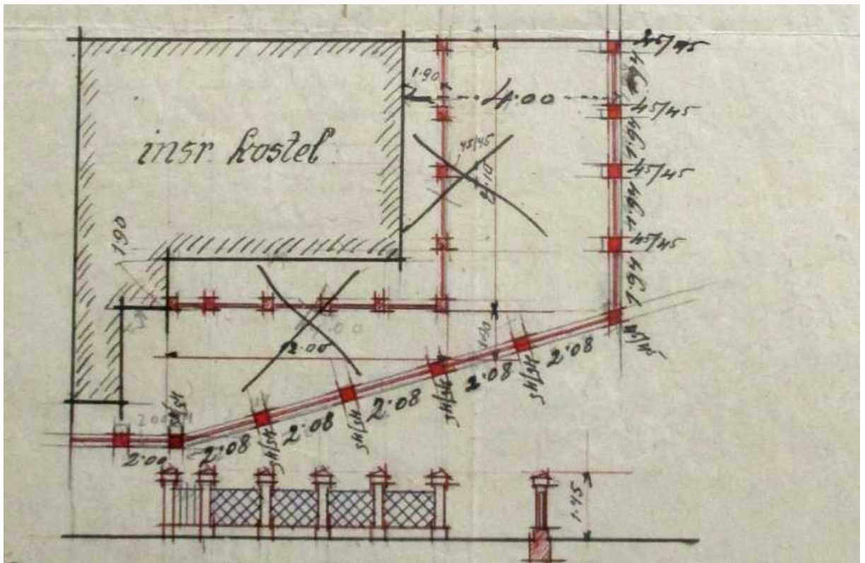
Obrázek č. 87: Stavební a konstrukční plán plotu, který byl okolo prostranství synagogy vztyčen v roce 1922
