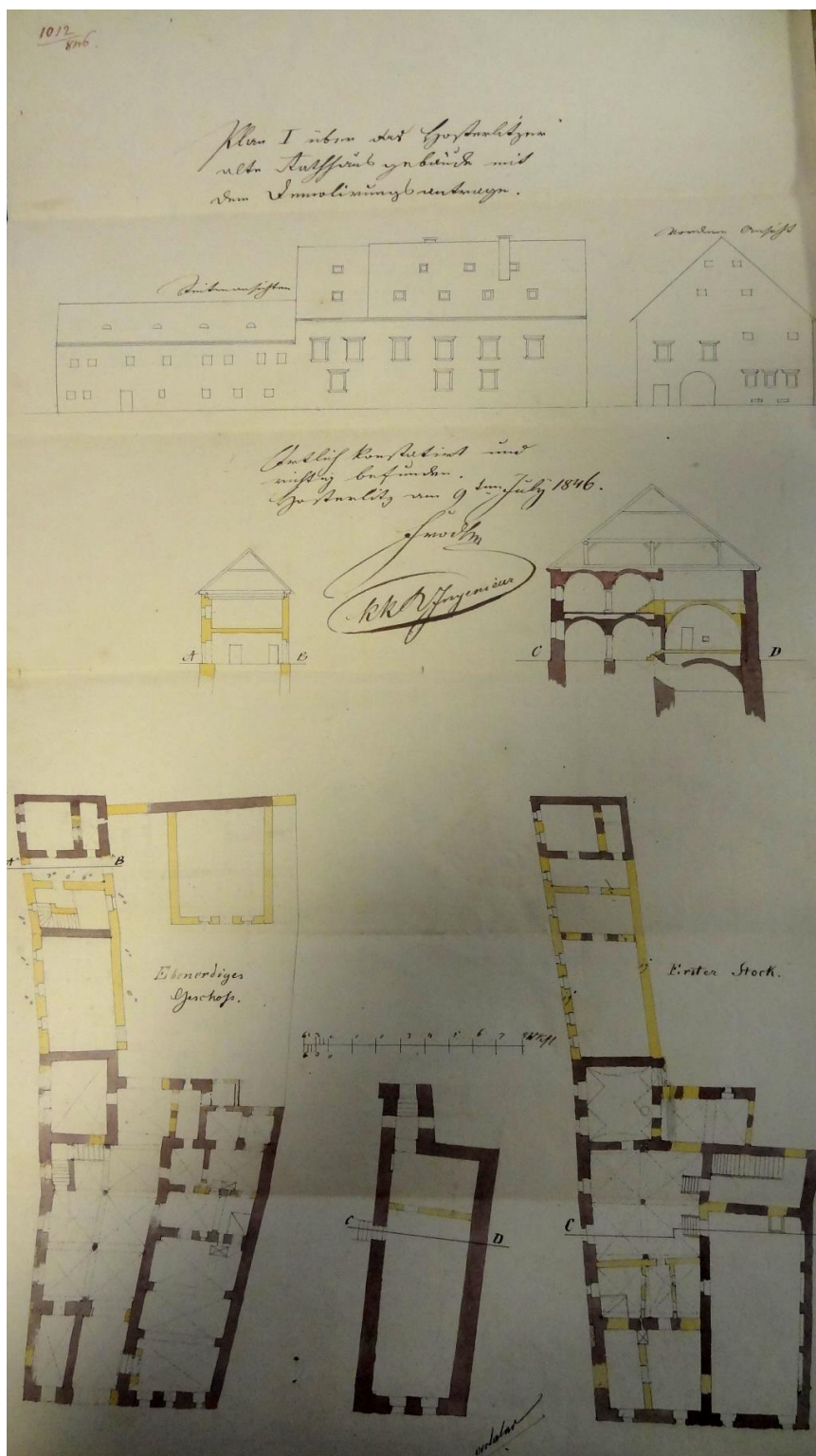
Příloha č. 48: Plán zachycující hostěradickou radnici v roce 1846, kdy se uvažovalo o její demolici a postavení nové. Její podobu i členění místností zachycuje vcelku přesně, povšimněme si především nestejně výšky podlah a pater i velmi hezky zachyceného prostoru obecního šenku (spodní patro v levé části i „sklep“ v části pravé v podélném řezu budovou).
